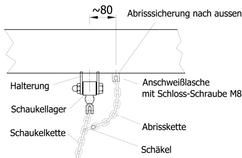
Detail Abrissicherung
